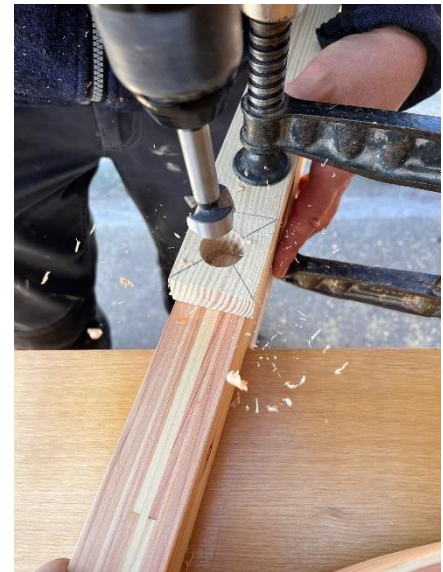
Abbildung 33 Loch bohren
