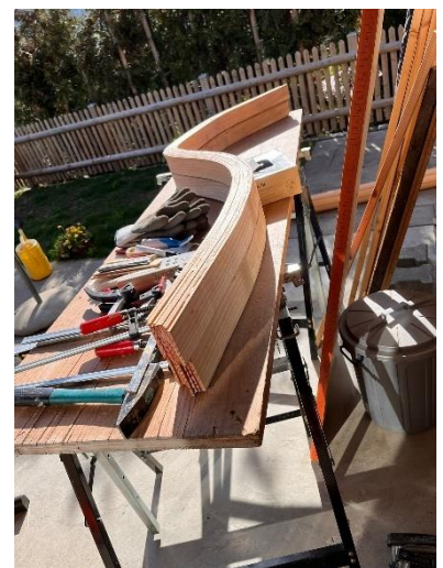
Abbildung 28 Gebogenes Holz
