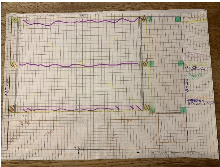
Abbildung 14 Skizze Podest von oben
